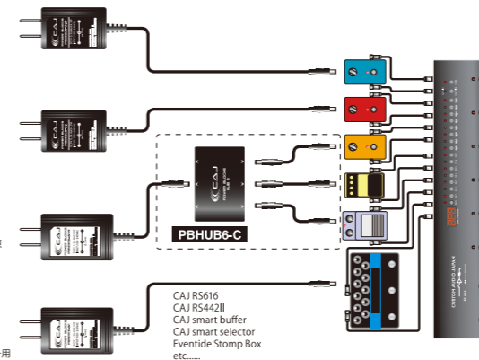
従来のパワーサプライを使用したシステム
